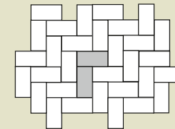
Verlegebeispiel 2 Bedarf pro m 2 = 68 Stück
